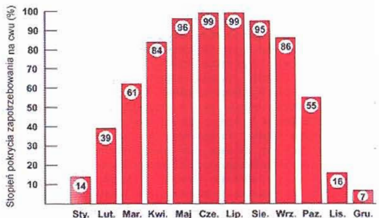
Szacunkowy stopień pokrycia zapotrzebowania na podgrzewanie ciepłej wody użytkowej energią słoneczną przy wykorzystaniu prawidłowo dobranej i wykonanej instalacji
